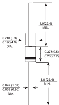
DO-201AD
